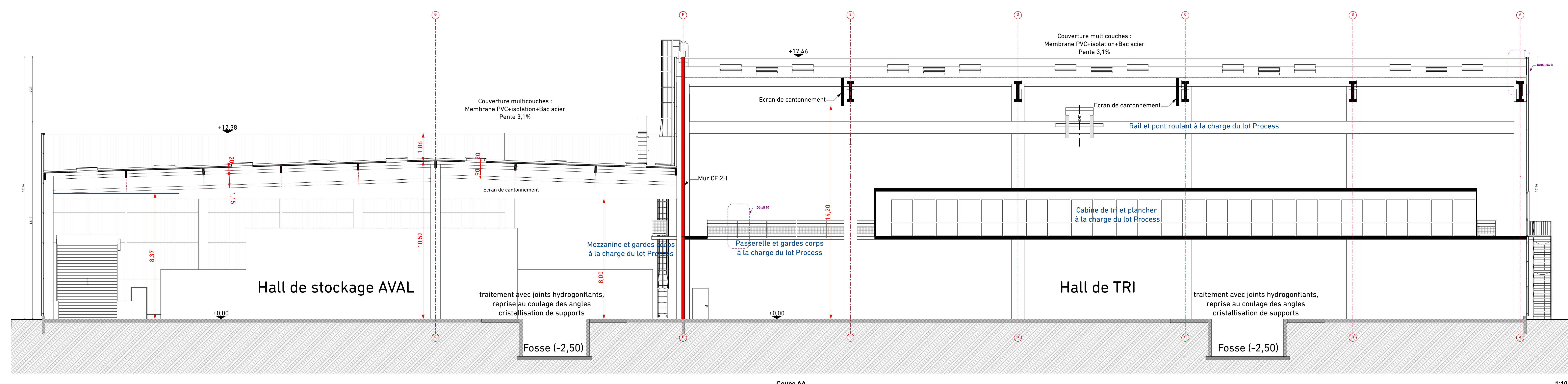
Coupe AA 1:100
