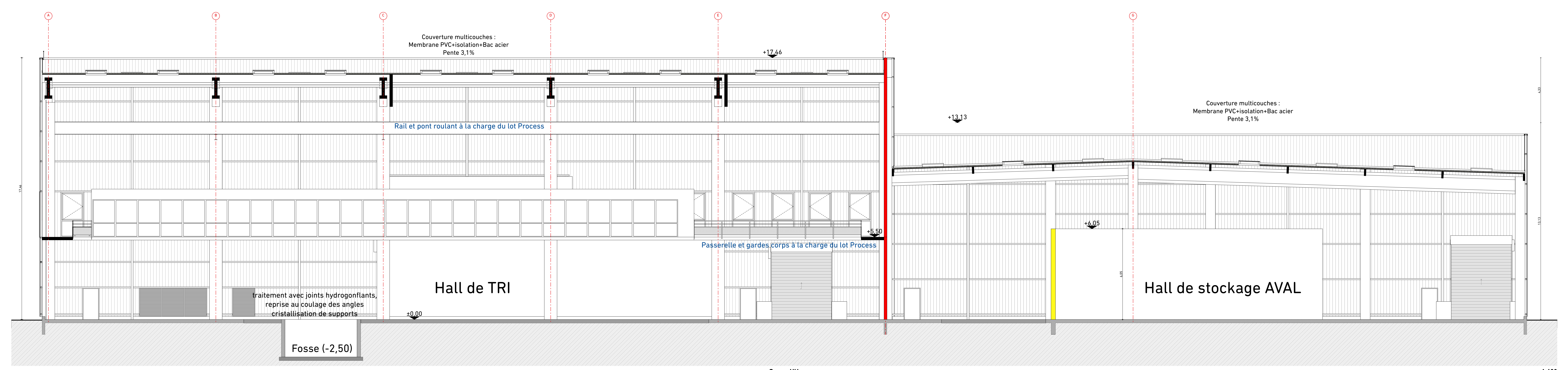
Coupe HH 1:100
